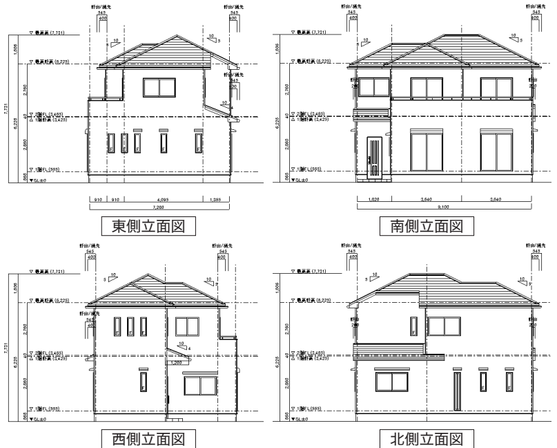
西側立面図
